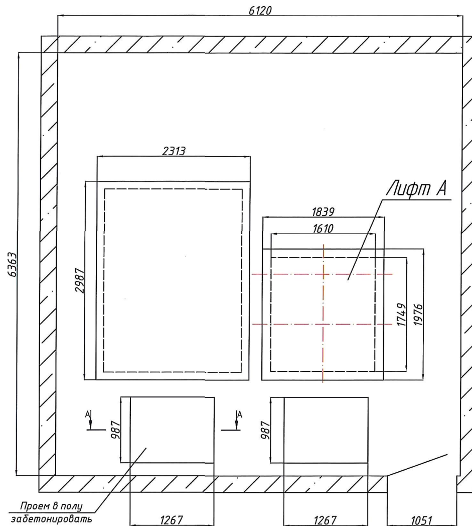
План машинного помещения
