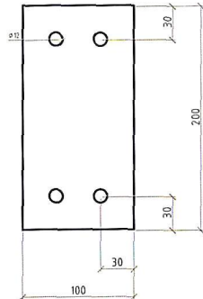
Закладная деталь М-6
