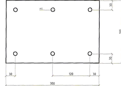
Закладная деталь М-10
