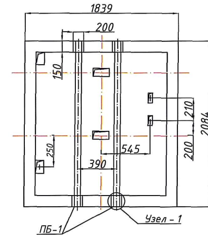
План расположения подлебедочных балок на перекрытии лифтовой шахты
