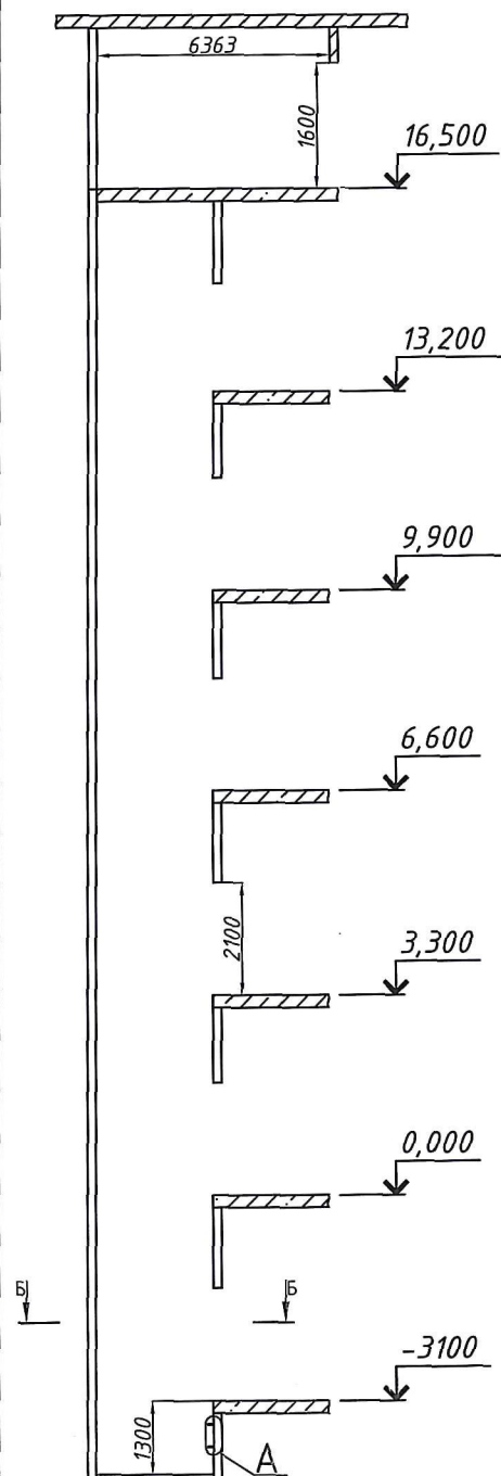
Разрез шахты лифта А
