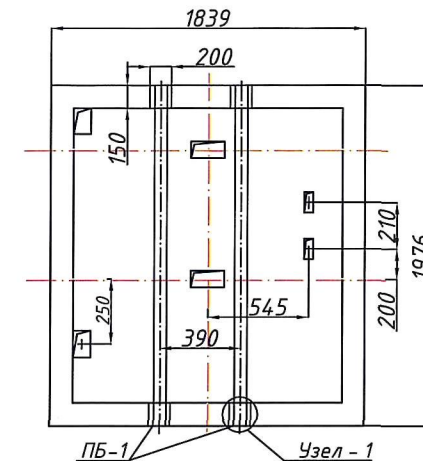
План расположения подлестничных балок на перекрытии лифтовой шахты
