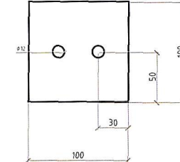
Закладная деталь М-10
