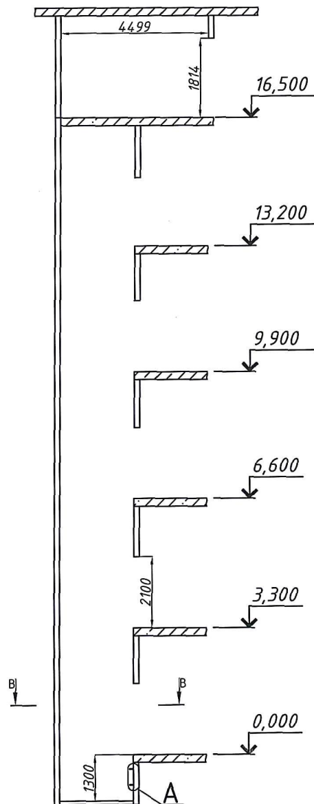
Разрез шахты лифта В
