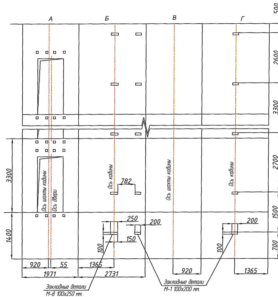
План шахты лифта Б
