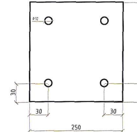
Закладная деталь М-9
