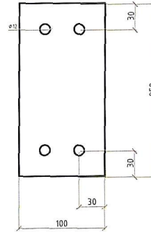
Закладная деталь М-8
