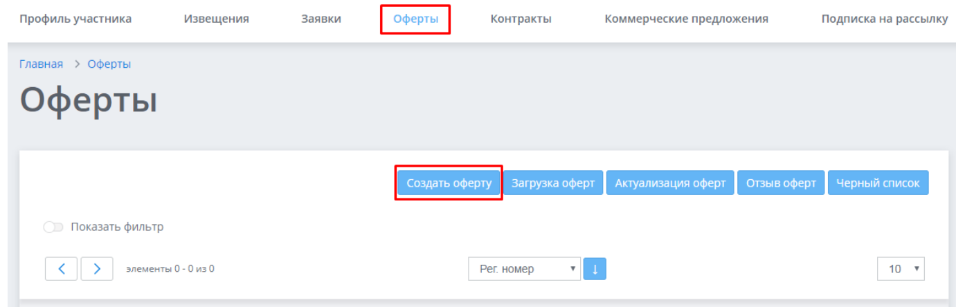
Рисунок 13. Создание offerты
