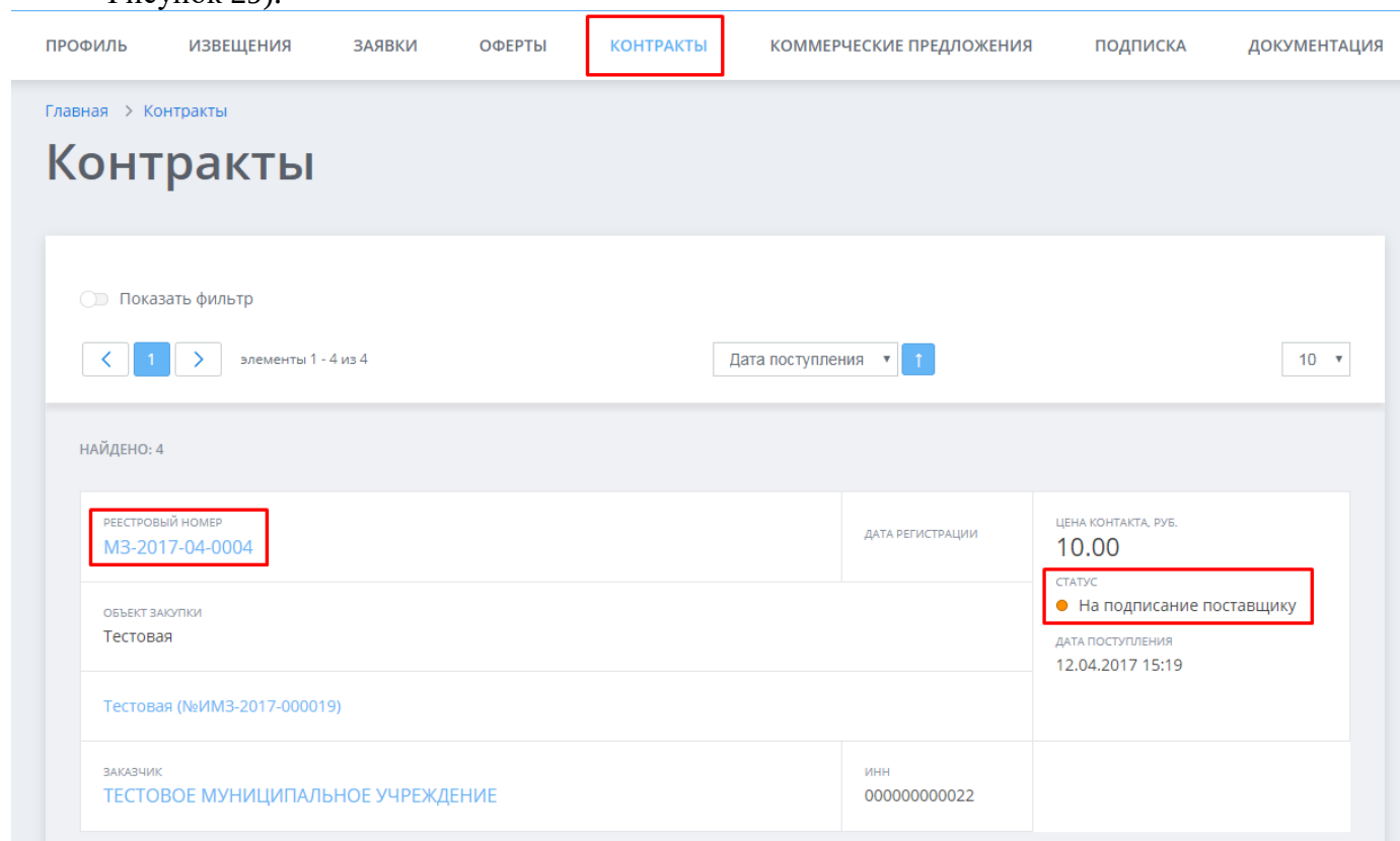
Рисунок 29. Заключение контракта
