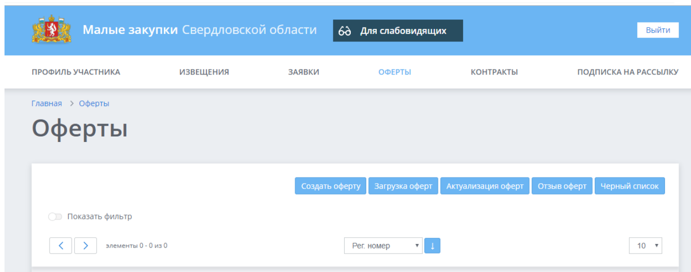
Рисунок 12. Оферты
