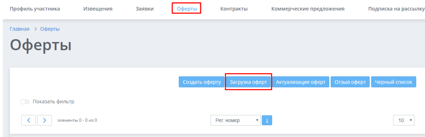
Рисунок 19. Загрузка оферт
