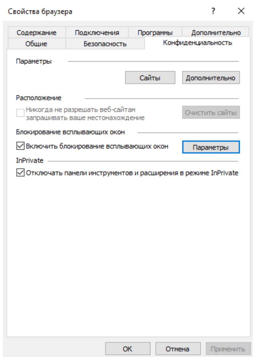
Рисунок 2. Вкладка Конфиденциальность
